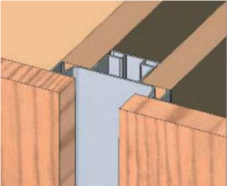
PRIKAZ MONTAŽE VERTIKALNOG PROFILA
