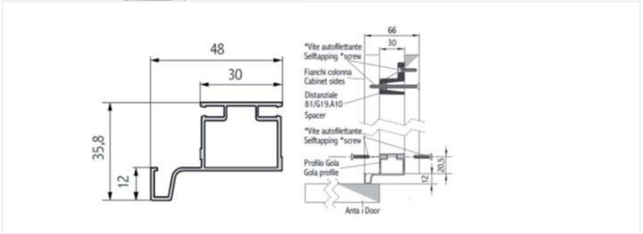
PRIKAZ MONTAŽE VERTIKALNOG PROFILA
