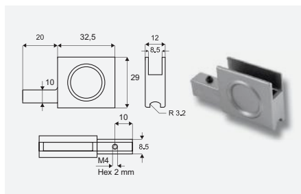
Br. artikla Opis artikla 2220228 Ručkica za klizna staklena vrata JM kom
