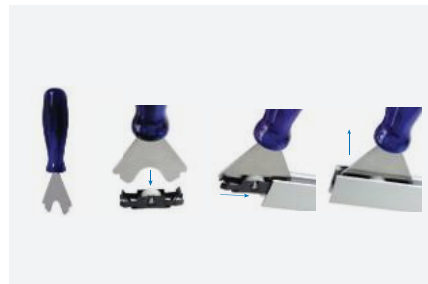
Br. artikla Opis artikla 2220231 Ručni alat za ugradnju kotačića JM kom
