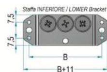
DONJI PRIHVATNIK
