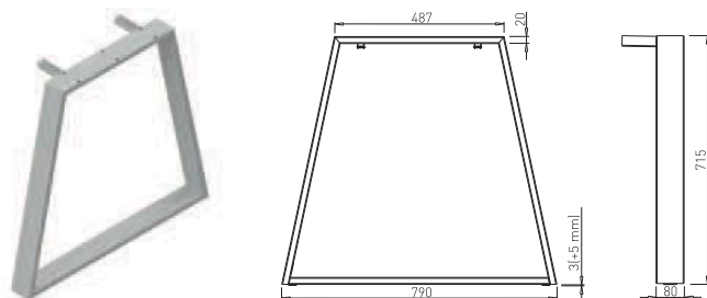
Noga model A-Leg, siva
