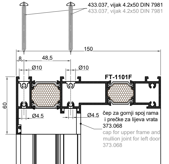
433.037, vijak 4.2x50 DIN 7981 433.037, screw 4.2x50 DIN 7981
