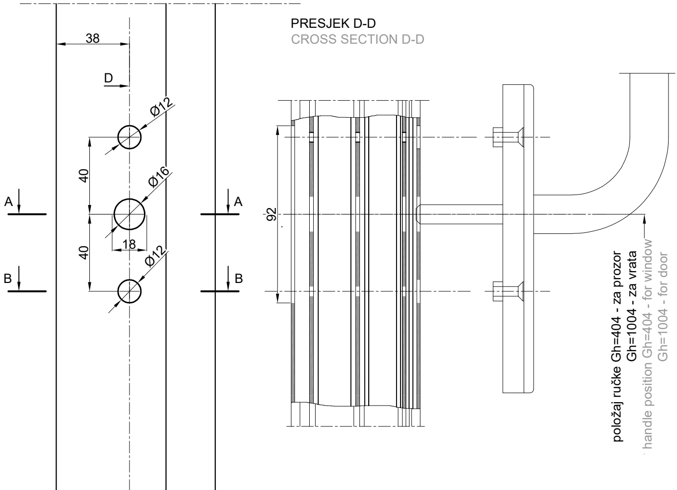
POGLED Obrada za vanjski rukohvatnik VIEW Processing for external finger grip
