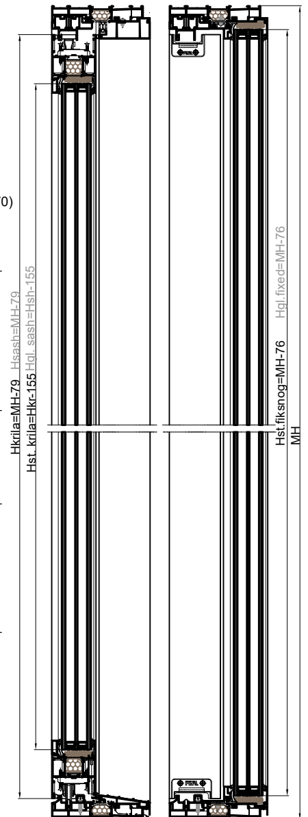
POMOĆNO KRILO AUXILIARY SASH GLAVNO KRILO BASIC SASH
