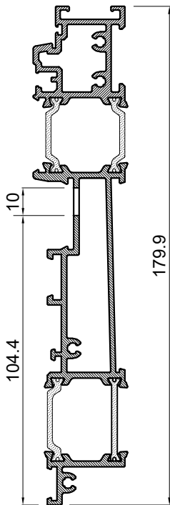
M 2:1 presjek A-A M 2:1 cross section A-A
