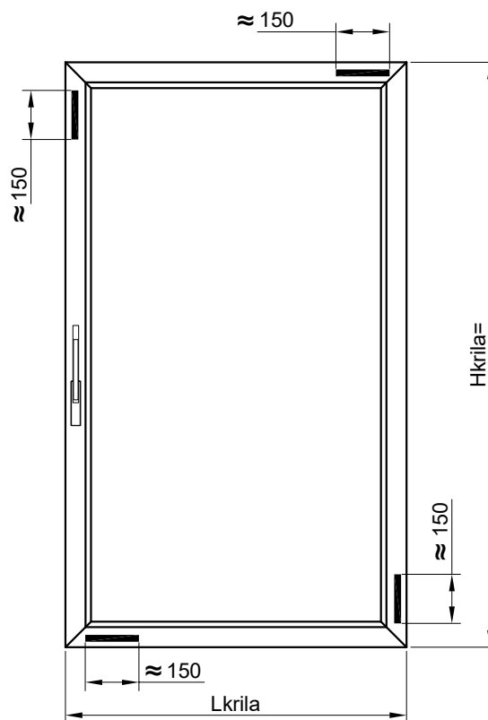
— Pozicija izrezivanja termo štapića (poliamida) na krilu \approx 150 mm
