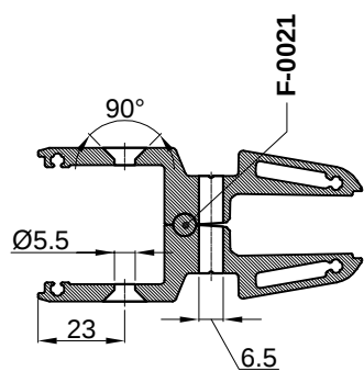
Presjek A-A
