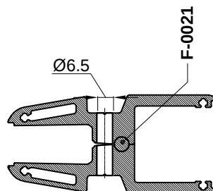
Presjek B-B
