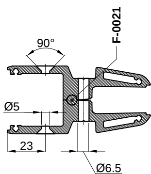
Presjek A-A
