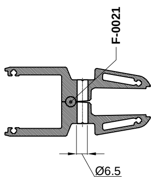
Presjek A-A
