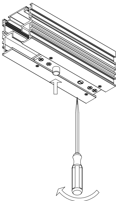
1. Podizanje trna zbog nanošenja vrata
