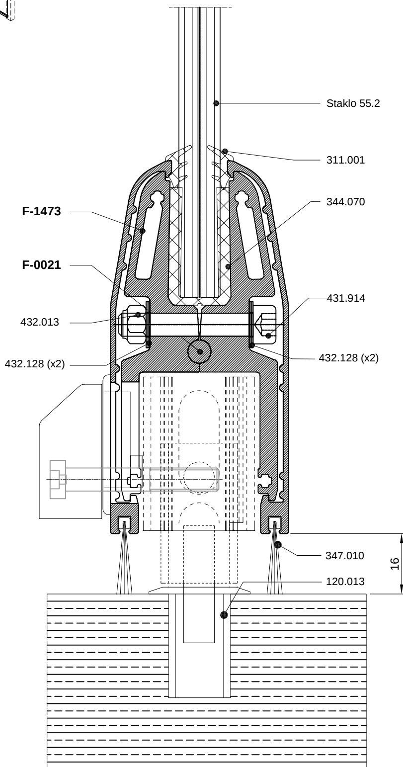
Klizna krila prvo i zadnje presjek - dolje
