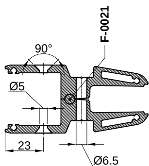
Presjek A-A
