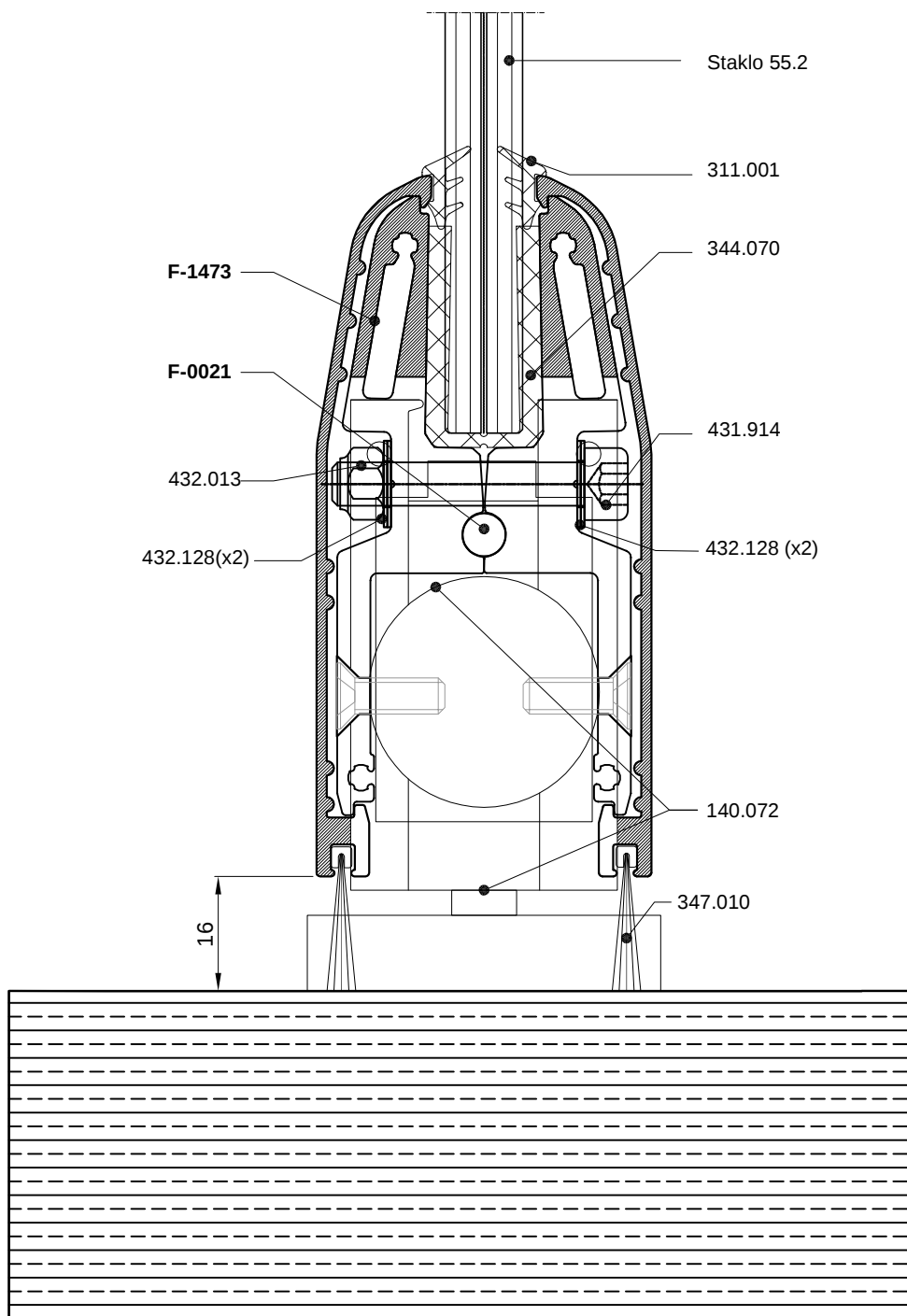
Mimokretna vrata presjek dolje automat u krilu - 140.072
