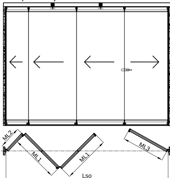
Tip otvaranja 3-1
