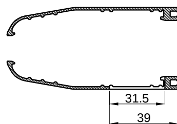
Presjek C-C
