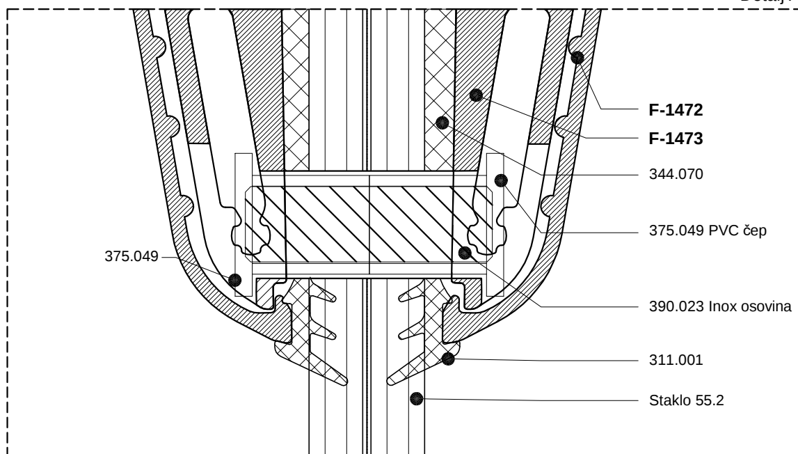
Detalj A
