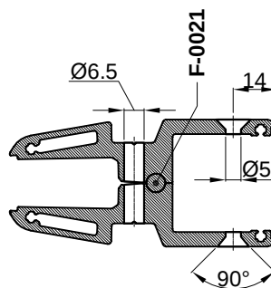
Presjek B-B
