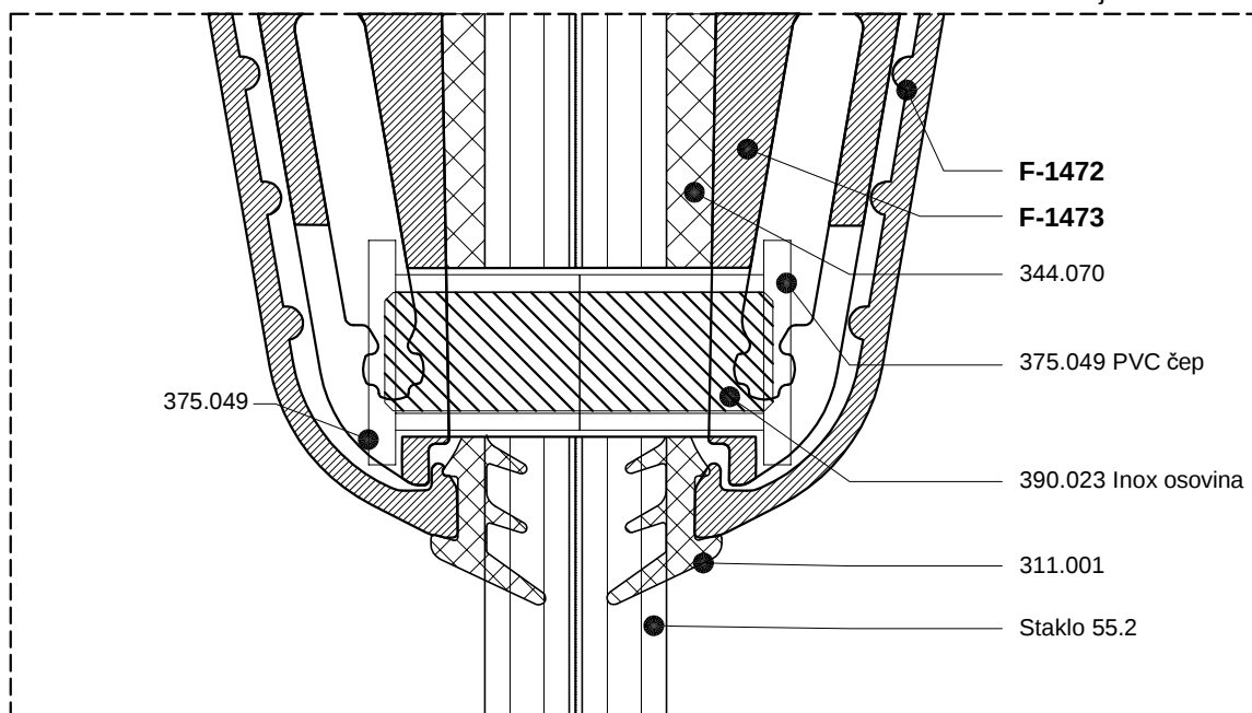
Detalj A
