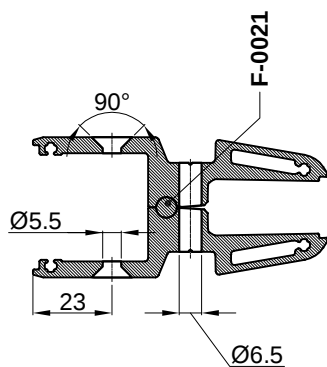
Presjek A-A
