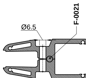
Presjek B-B
