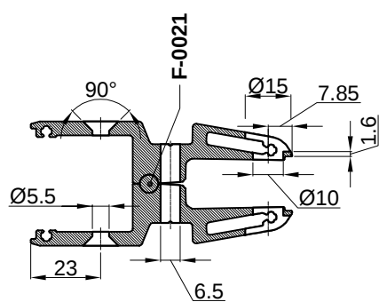
Presjek A-A
