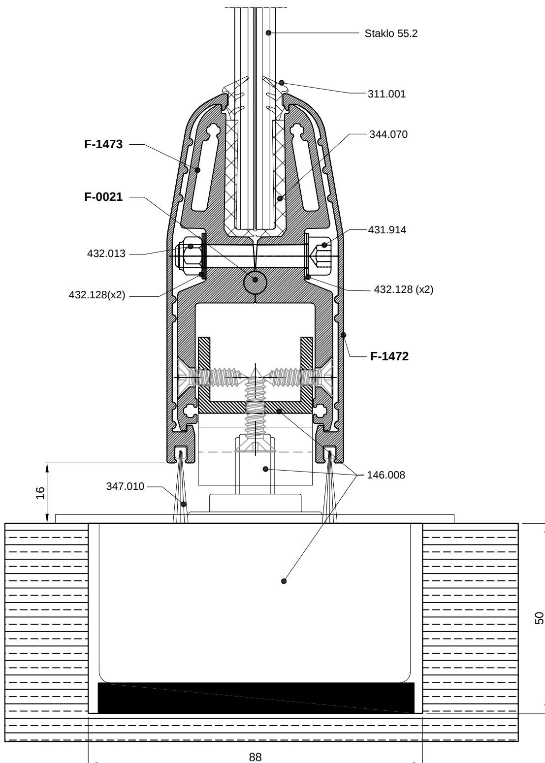
Mimokretna vrata presjek dolje automat u podu - 146.008
