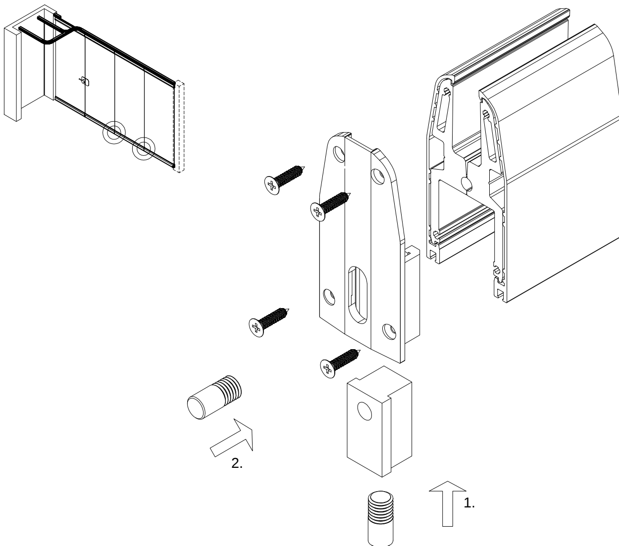
Zatvoreni položaj
