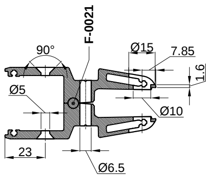
Presjek A-A
