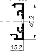
Presjek A-A M1:2 F-1660
