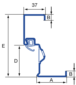
DryFix dovratnik
