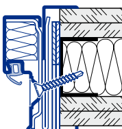
Dijagonalno pričvršćenje Montažni zid F90A
