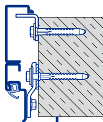
Skrivena montaža Cigleni zid
