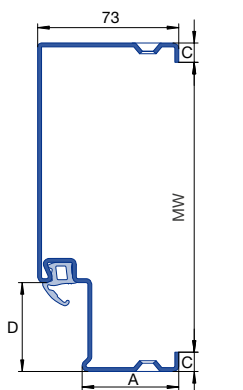
Obuhvatni dovratnik B73 za pregradne zidove
