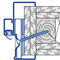
Dijagonalno pričvršćenje Montažni zid F90B
