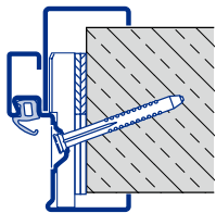
Dijagonalno pričvršćenje Cigleni zid / Neožbukani beton
