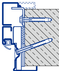
Dijagonalno pričvršćenje Neožbukani zid / beton
