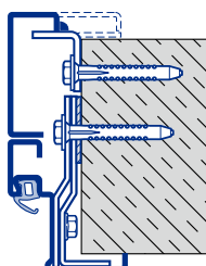
Ugradnja u otvor Cigleni zid
