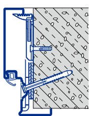
NOVO. Dijagonalno pričvršćenje Porobeton do MW 450
