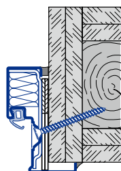
Dijagonalno pričvršćenje Montažni zid F90B
