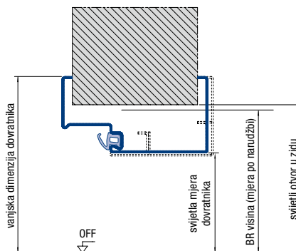
Dovratnik koji obuhvaća 4 strane (vrata) BR širina BR visina
