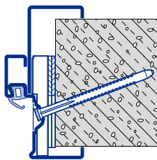
Dijagonalno pričvršćenje Porobeton
