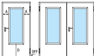
Ostakljenje slika 3
