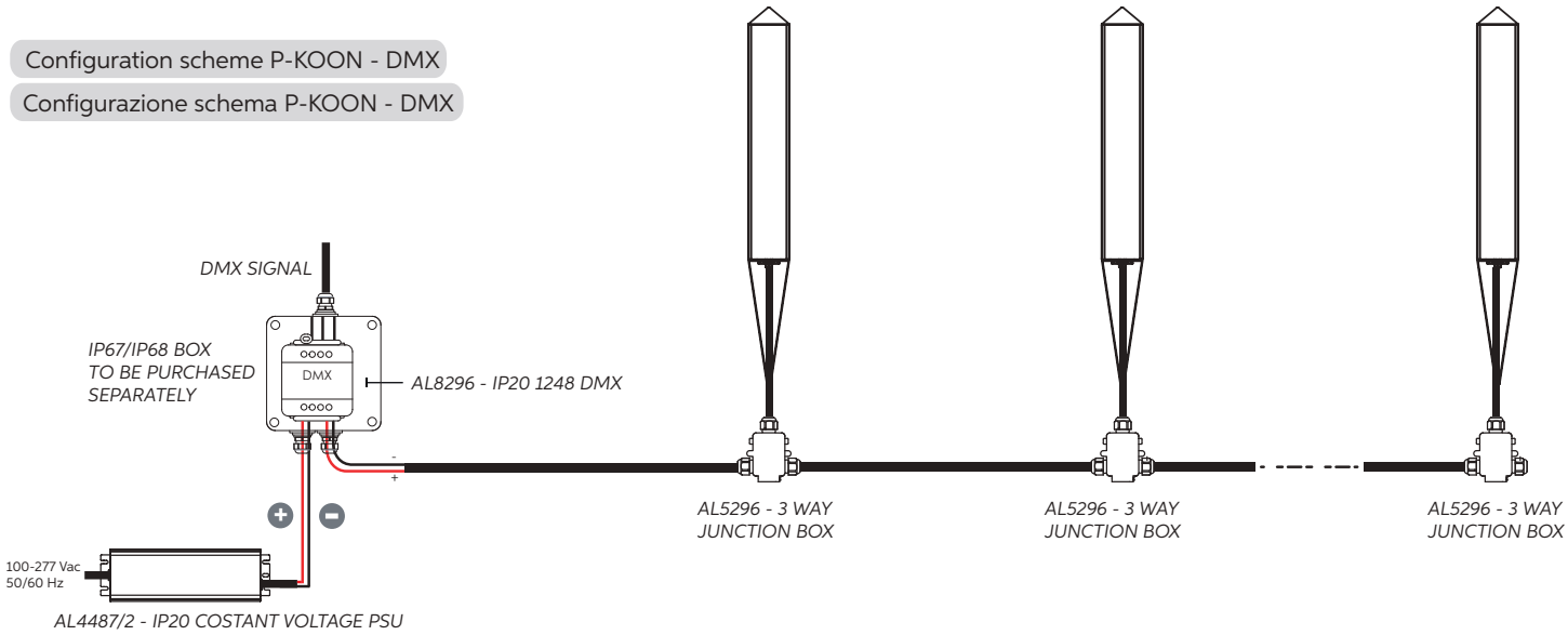
Configuration scheme P-KET - 0/1-10v Configurazione schema P-KET - 0/1-10V
