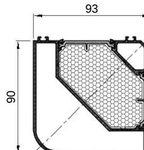
FT-0542F kg/m 2.398
