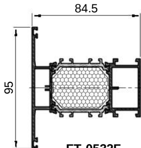
FT-0532F kg/m 1.875
