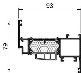
FT-0520F kg/m 1.743
