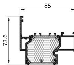
FT-0512F kg/m 1.671
