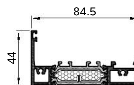
FT-0514F kg/m 1.248
