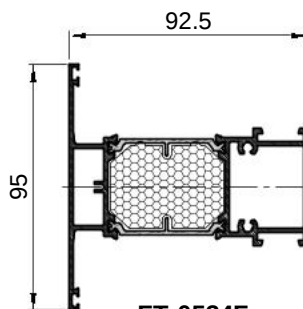
FT-0534F kg/m 1.913
