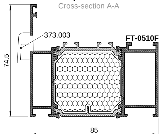
Presjek A-A Cross-section A-A
