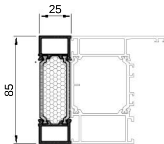
FT-0267F kg/m 1.036
