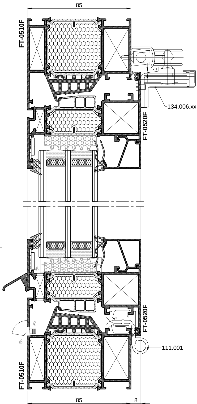
OTKLOPNI PROZOR - VENTUS s ručkom za visinu - (134.006.xx) TILT WINDOW - VENTUS with handle for height - (134.006.xx)
