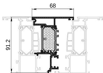
FT-0530F kg/m 1.563
